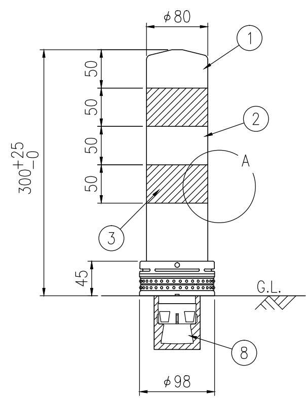
設置図 S=1/5
