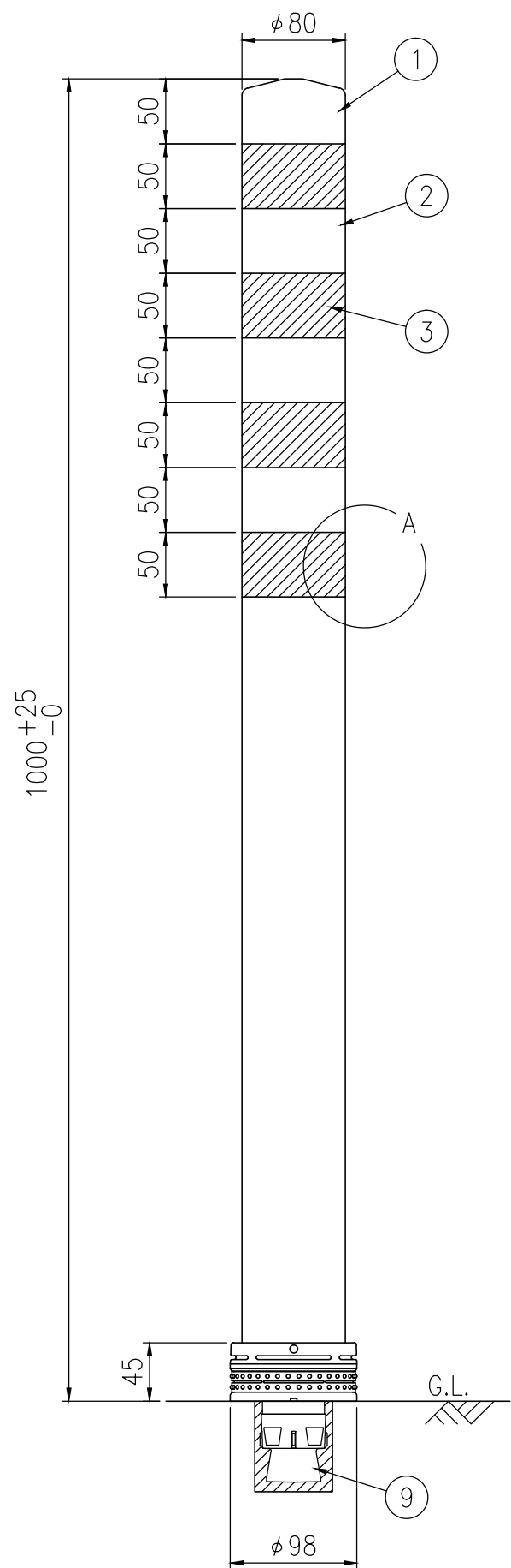
設置図 S=1/5
