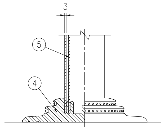
ベース部詳細図 S=1/4
