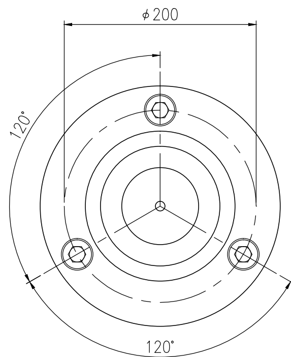
上面図 S=1/4
