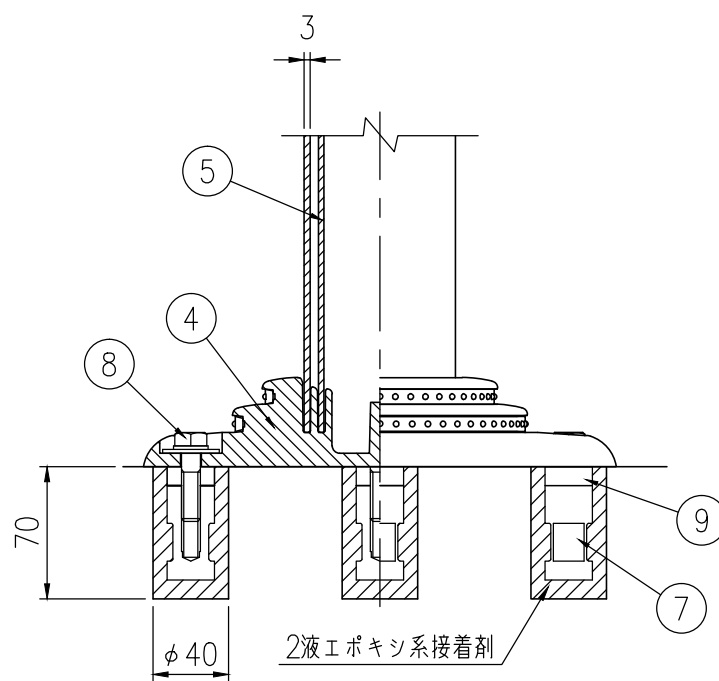
ベース部詳細図 S=1/4
