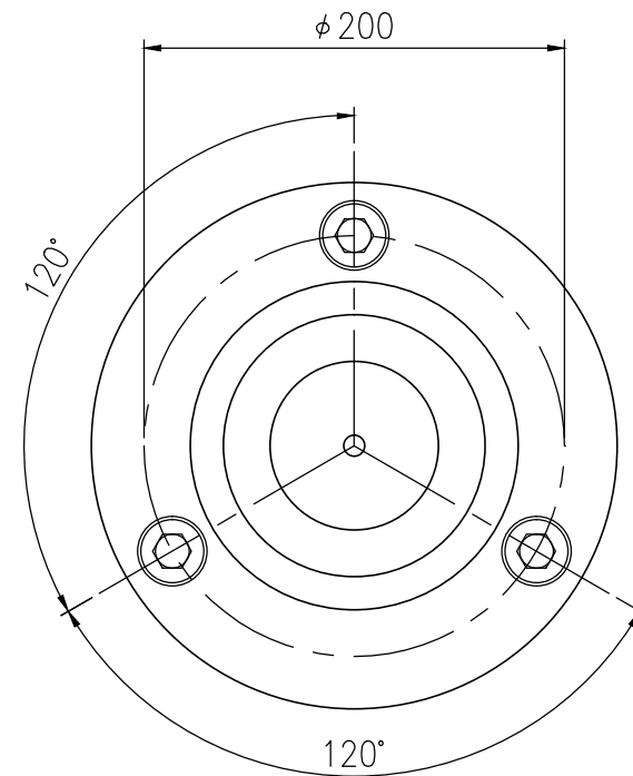
上面図 S=1/4
