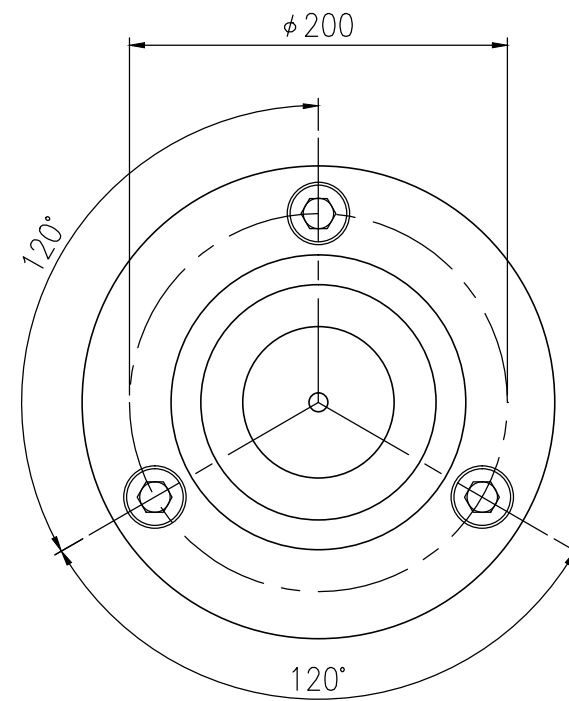
上面図 S=1/4
