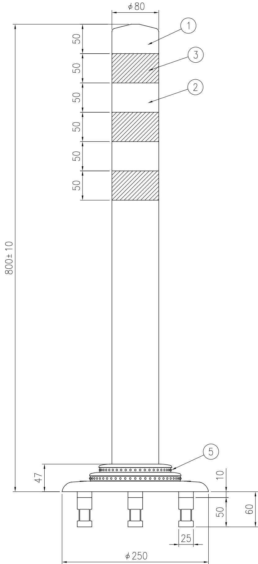
姿図 S=1/4
