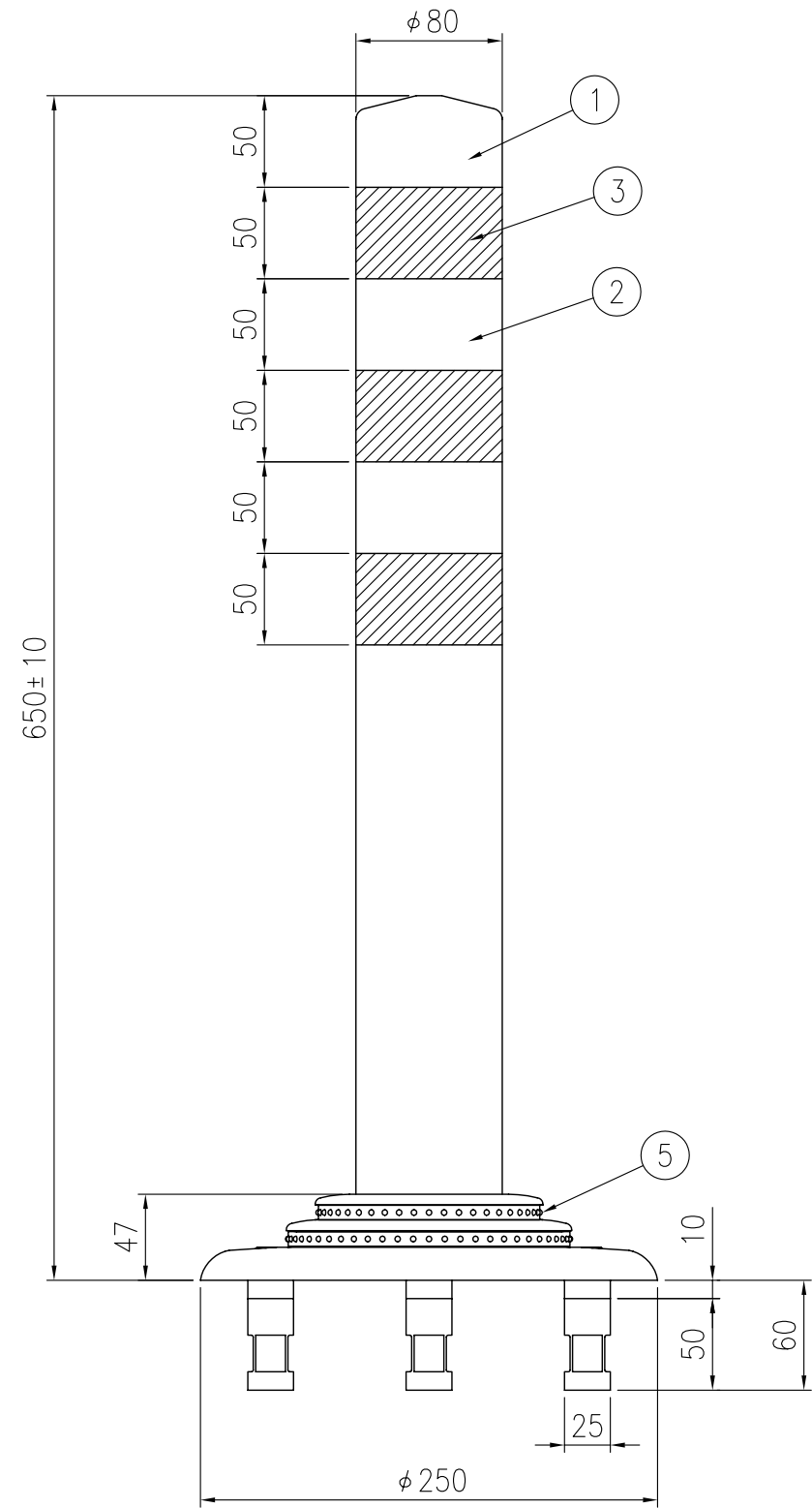
姿図 S=1/4
