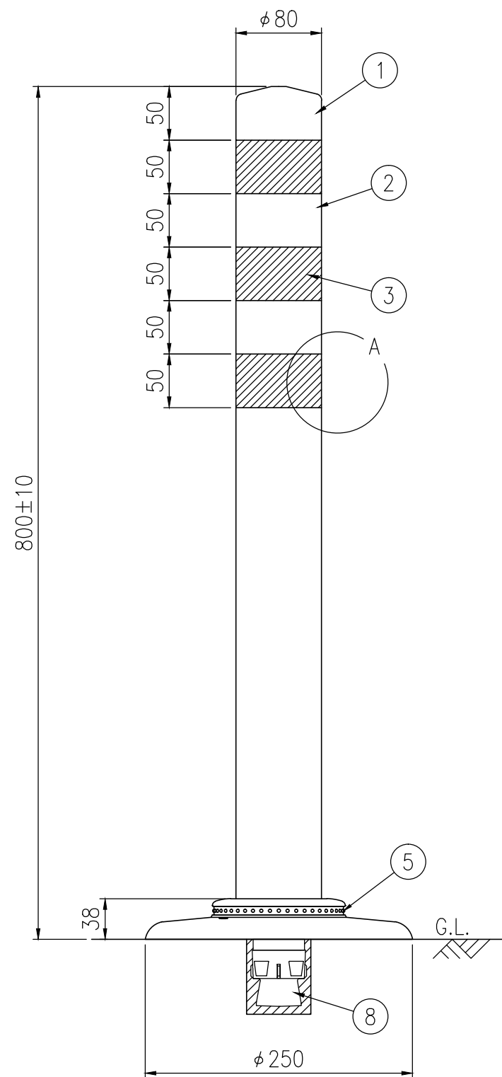
設置図 S=1/5
