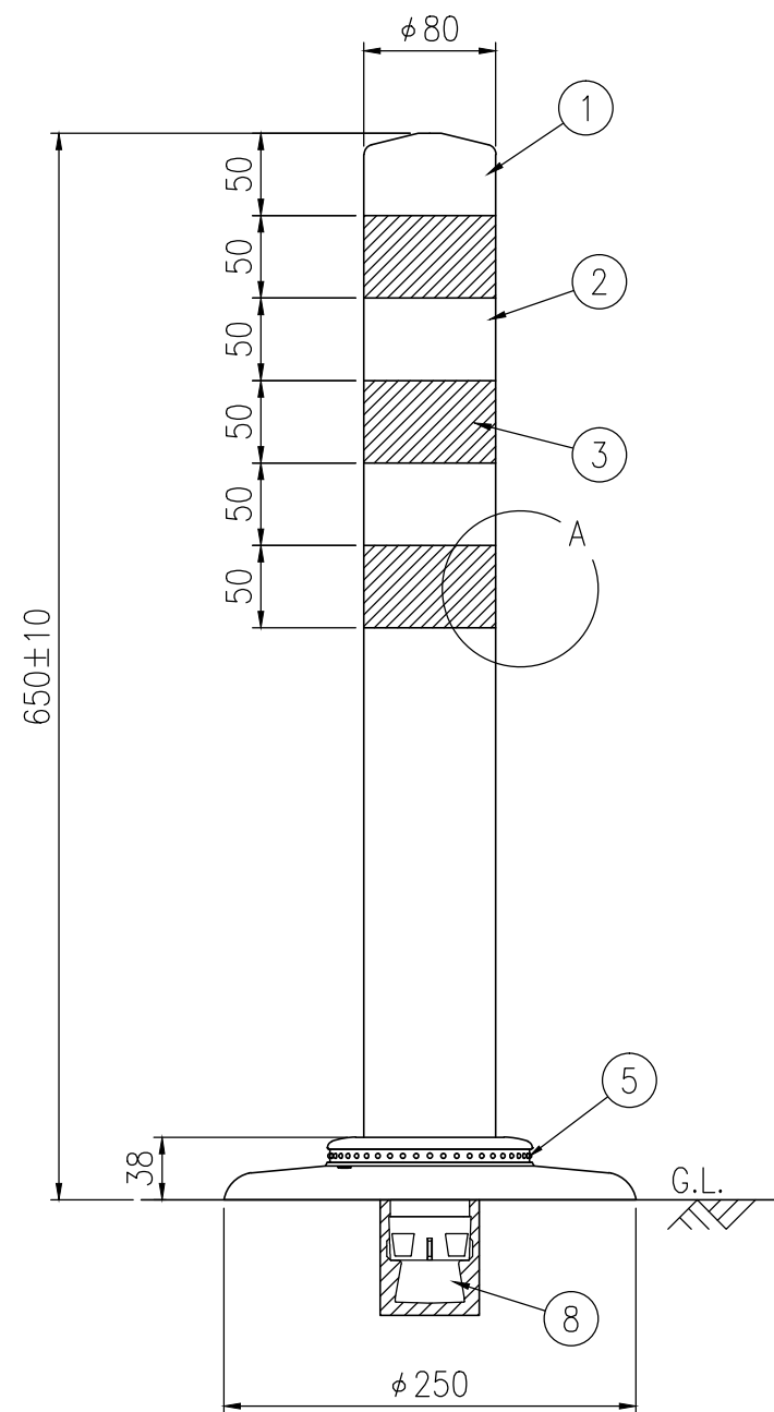
設置図 S=1/5
