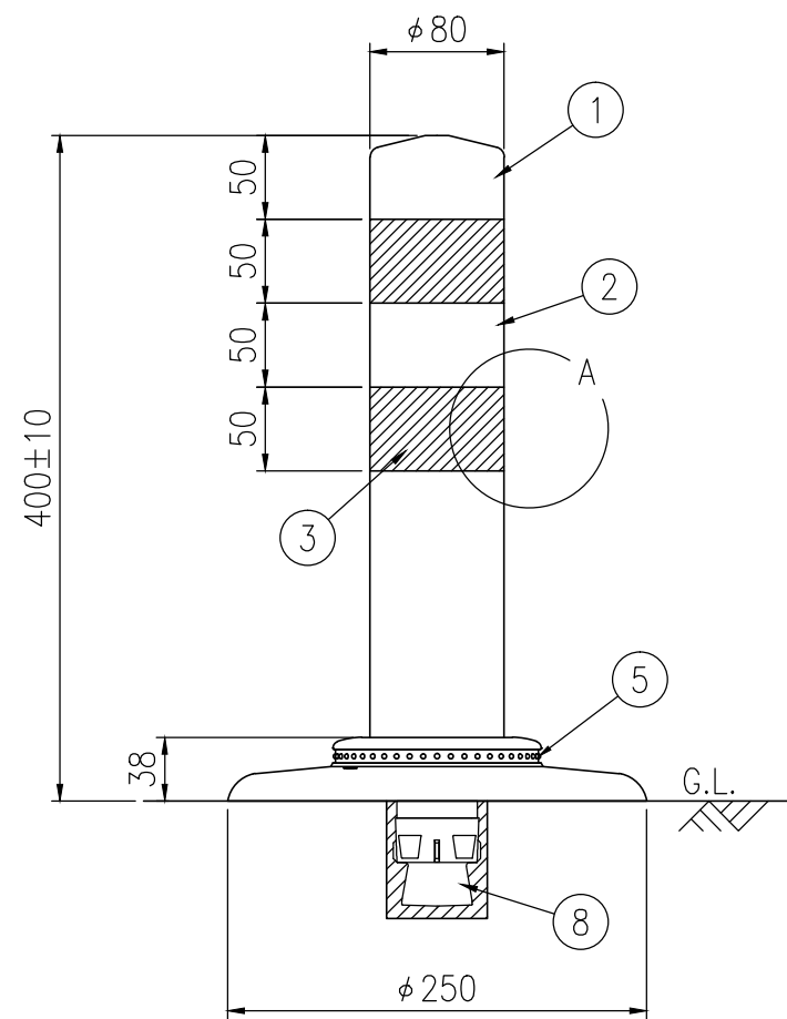
設置図 S=1/5
