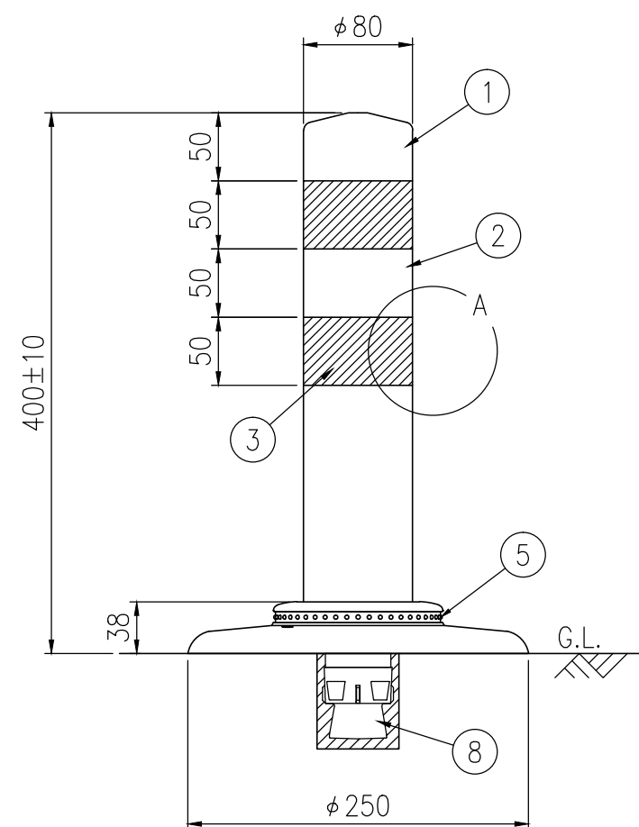
設置図 S=1/5
