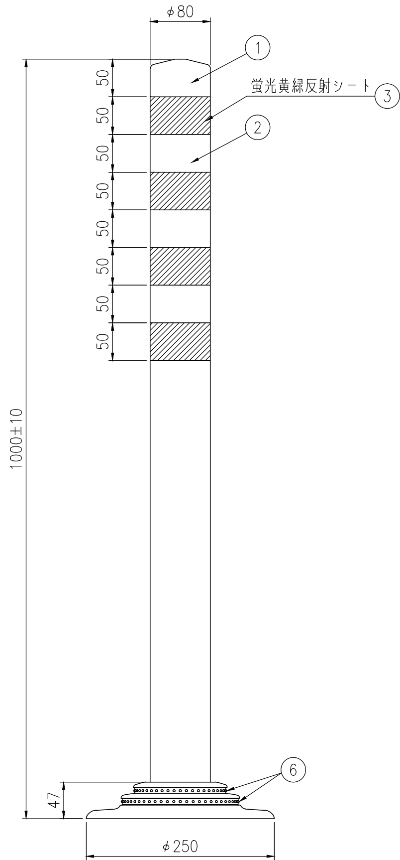
姿図 S=1/5
