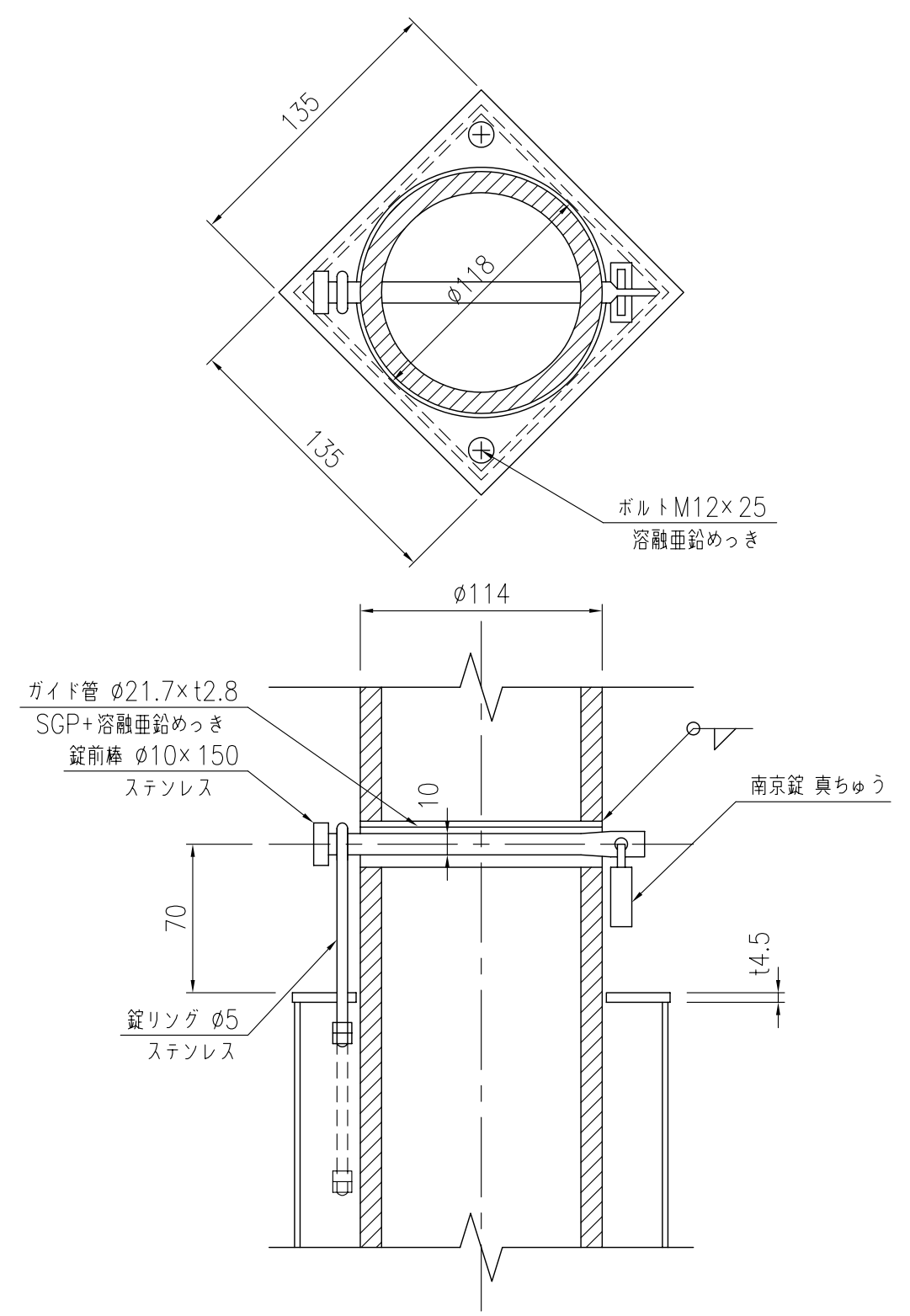
カギ部取付詳細図
