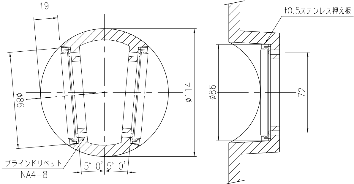
反射板取付部詳細
