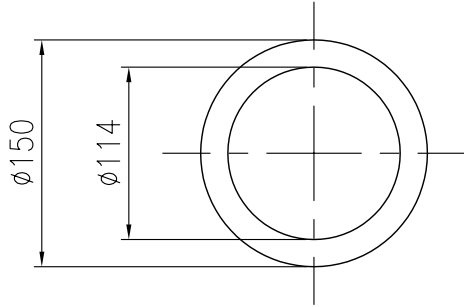
平面图
