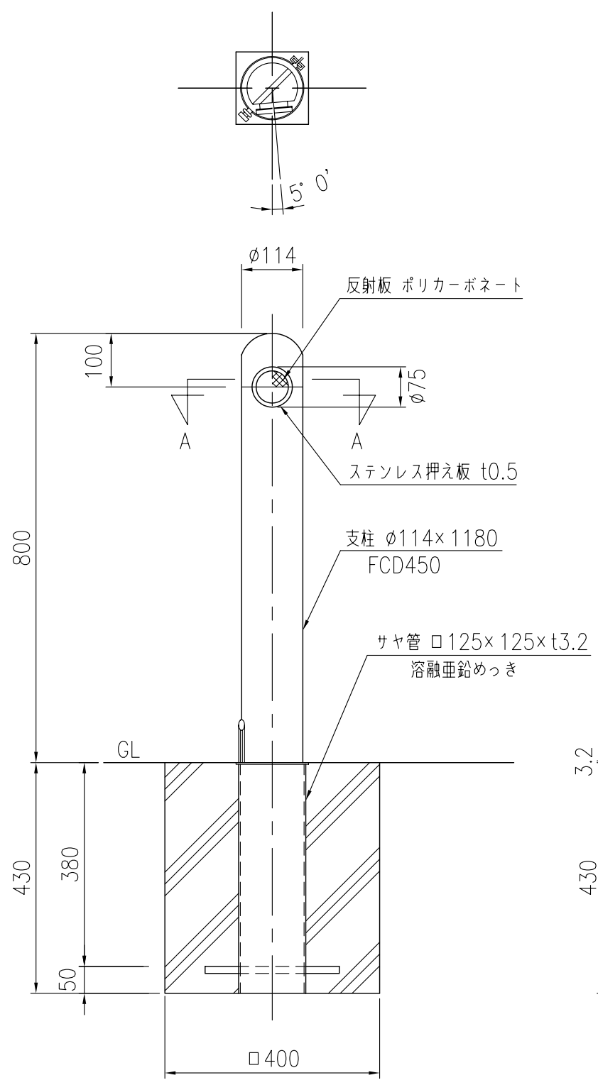
A-A断面
