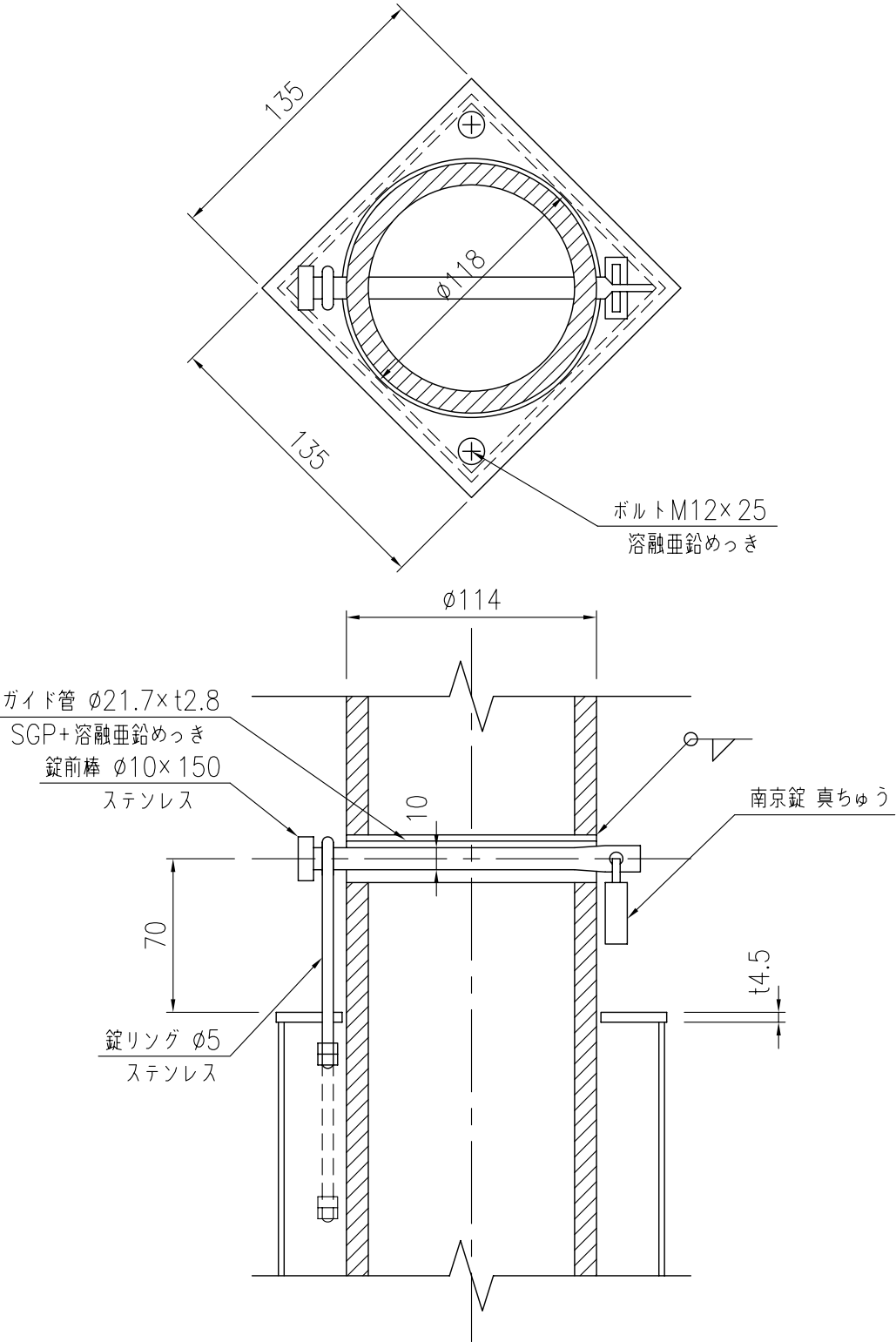
カギ部取付詳細図
