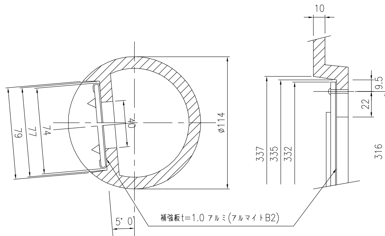
反射板取付部詳細
