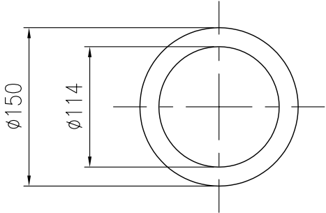
反射板取付部詳細
