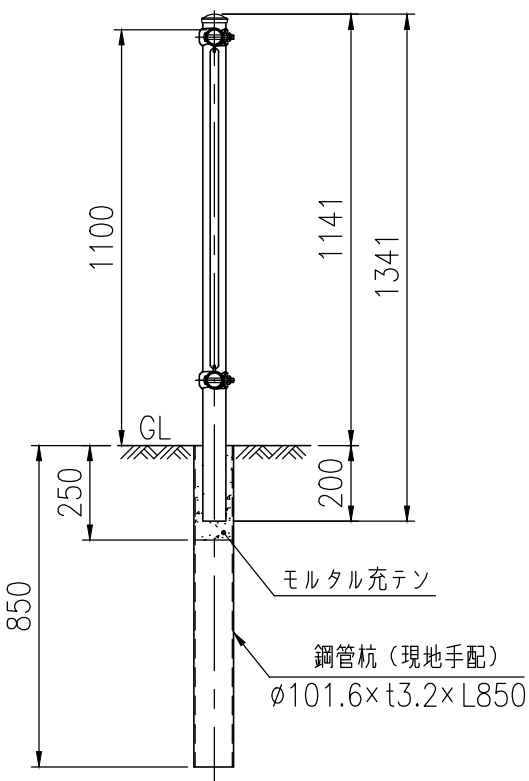
XTC-211W30(鋼管杭仕様)
