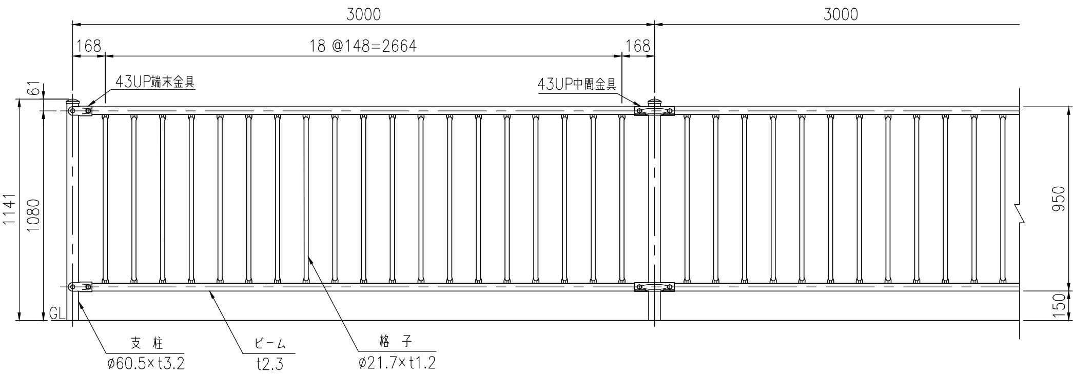
設置図 (1/20)
