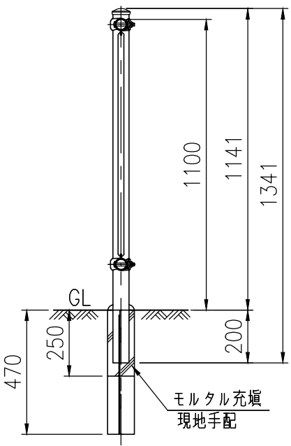
基礎杭 詳細図 (1/10)
