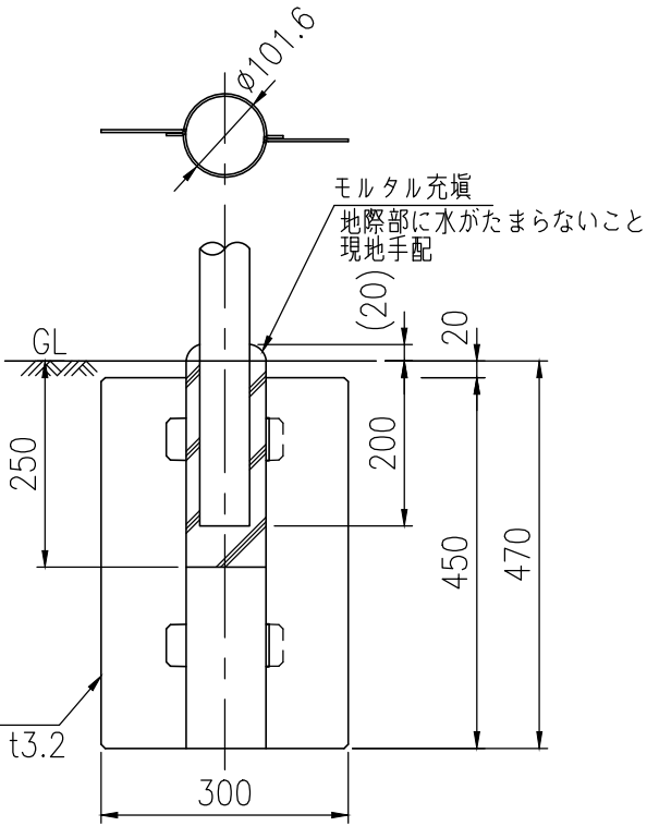
基礎杭 詳細図 (1/10)
