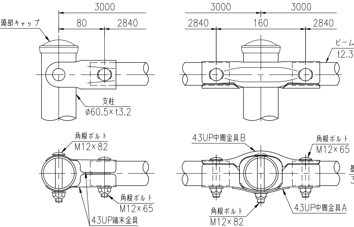
取付部詳細図 (1/4)
