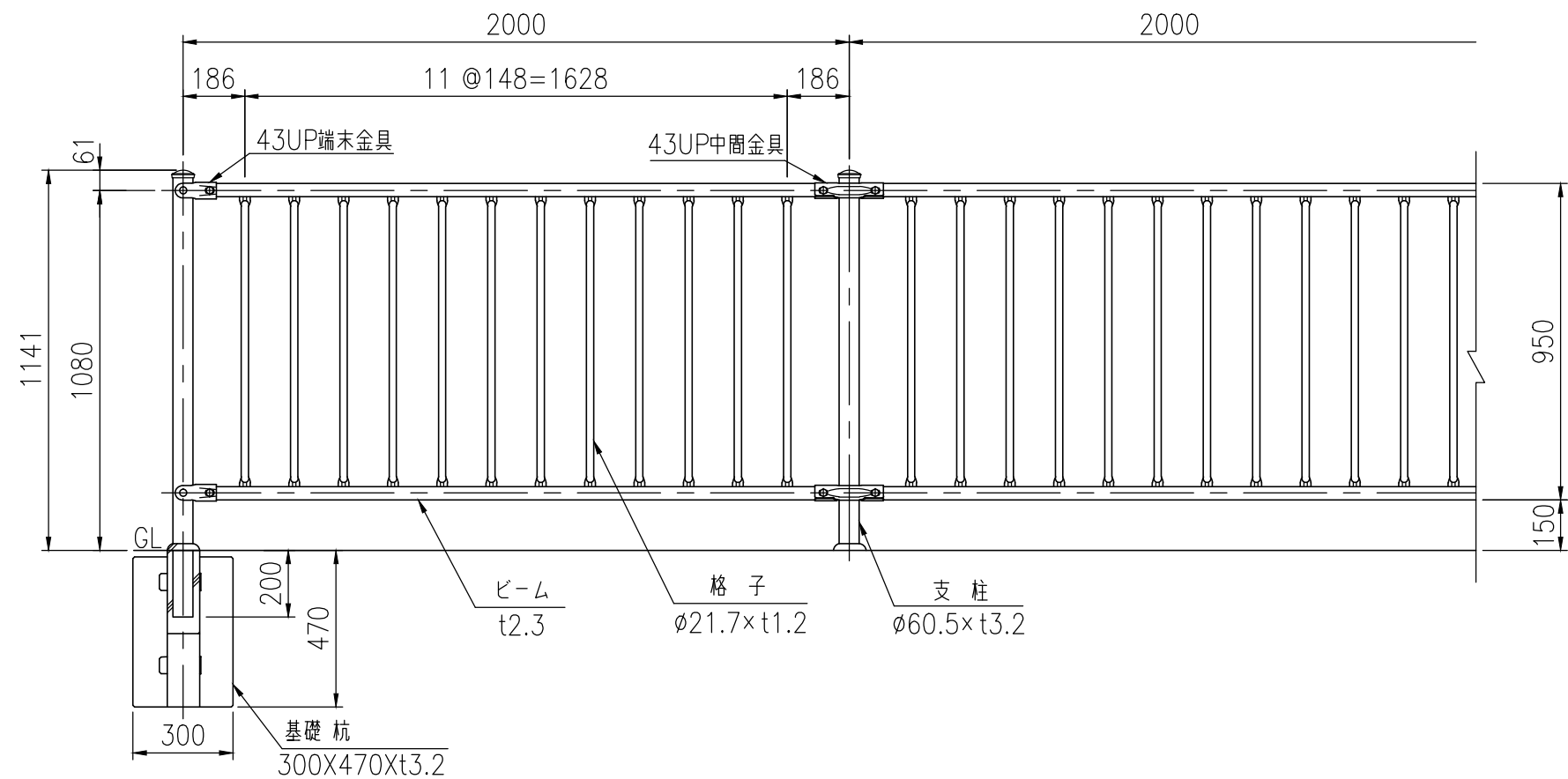
XTC-211W20(簡易基礎杭仕様)
