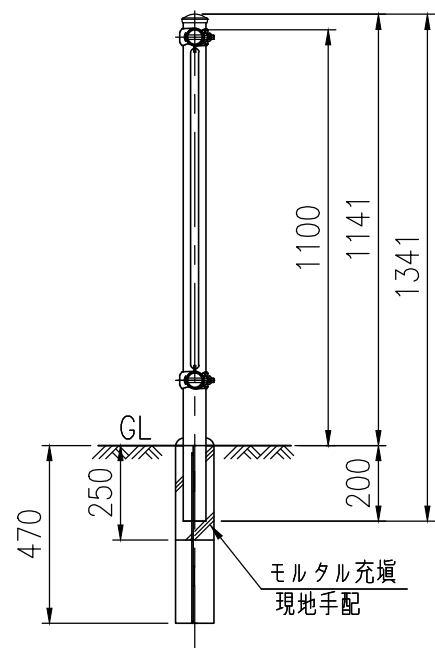
XTC-211W20(簡易基礎杭仕様)
