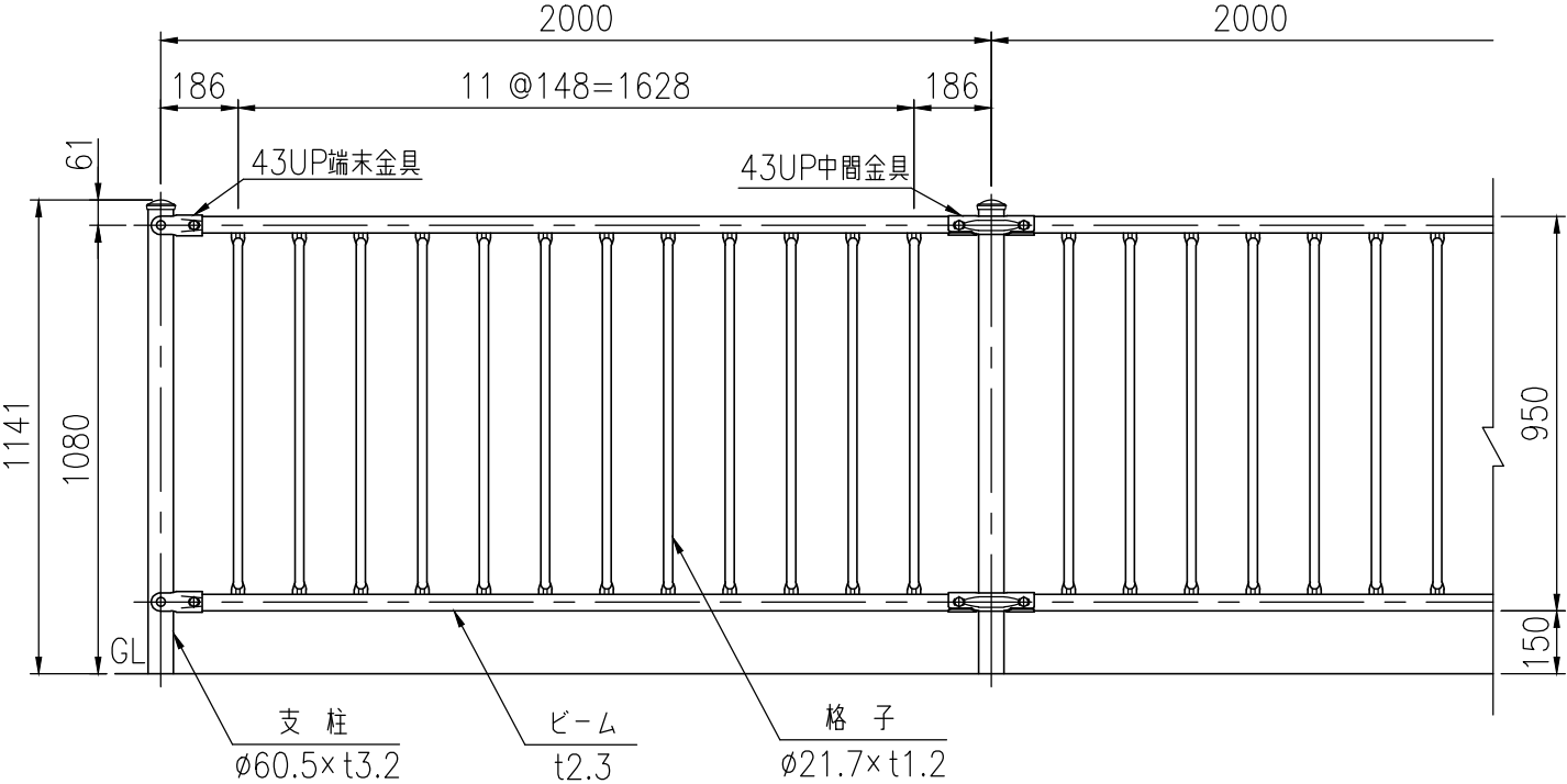
設置図 (1/20)
