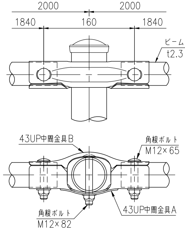
取付部詳細図 (1/4)
