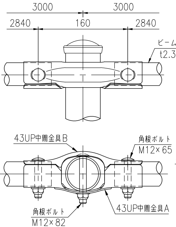
取付部詳細図 (1/4)
