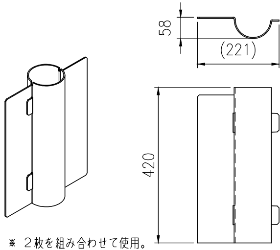
基礎杭 詳細図 (1/10)
