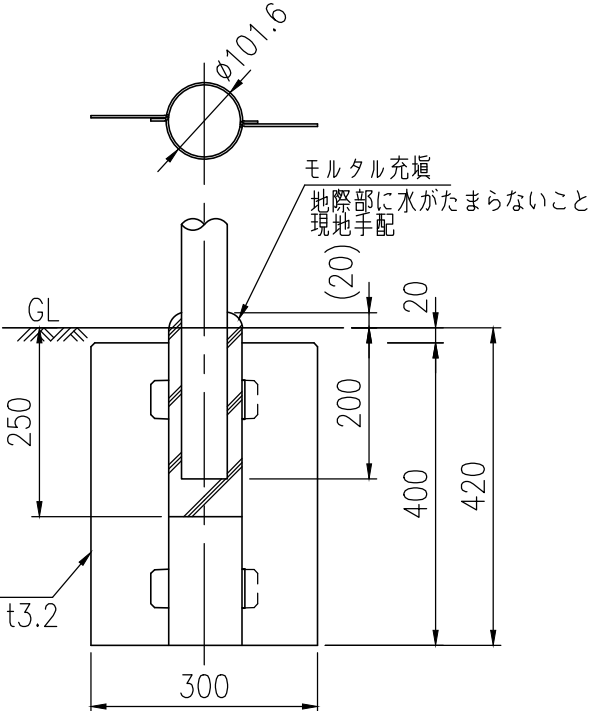
基礎部納まり 詳細図 (1/10)
