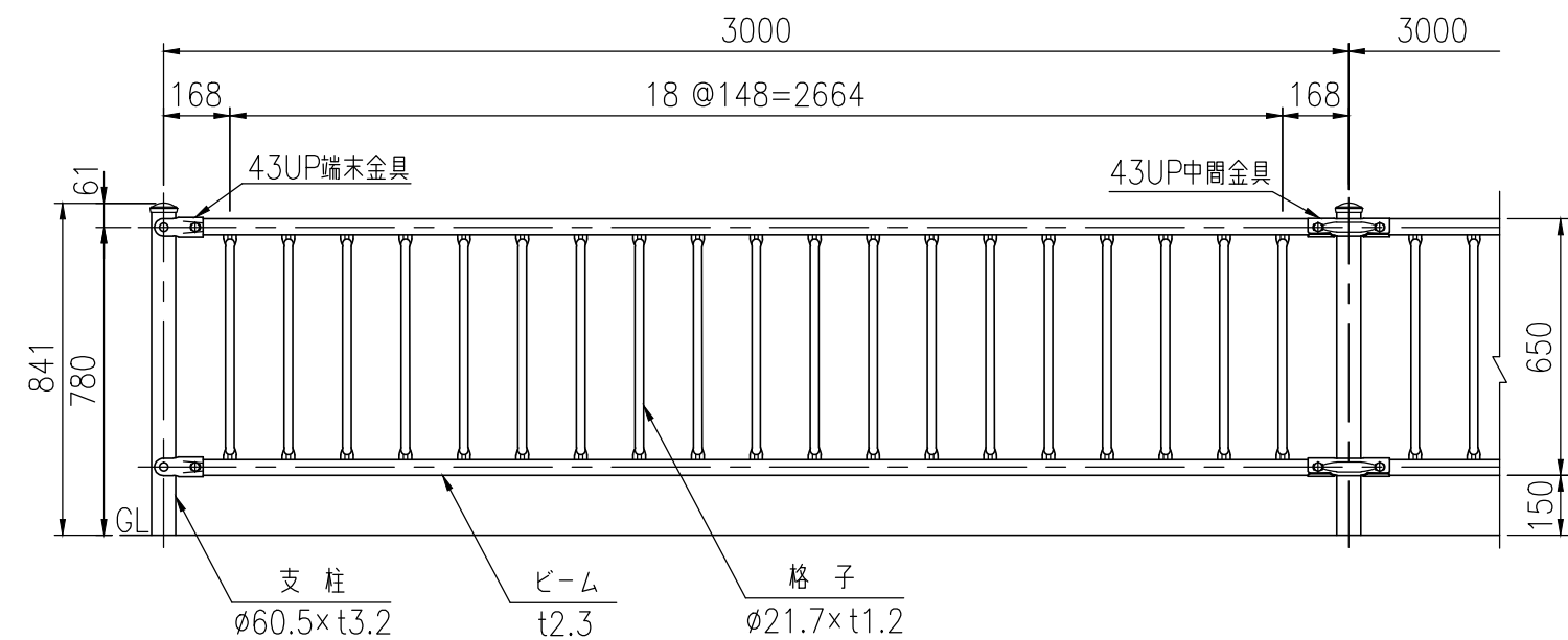
設置図 (1/20)
