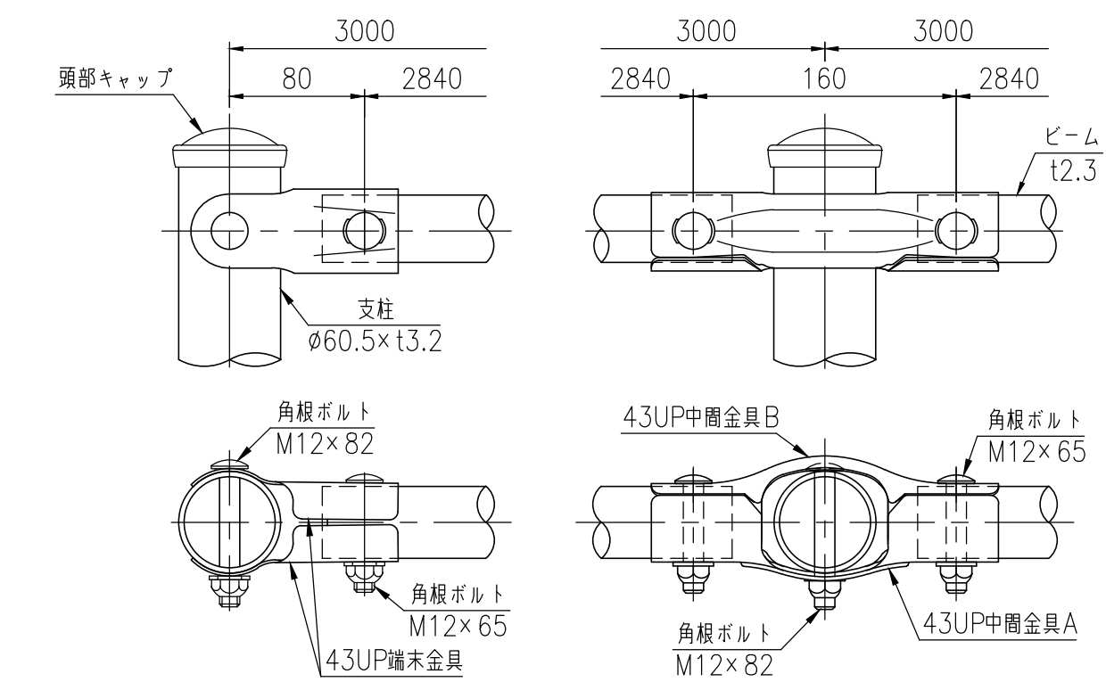
取付部詳細図 (1/4)
