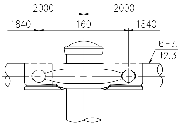
取付部詳細図 (1/4)
