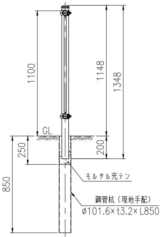
FXTC-211W30(鋼管杭仕様)
