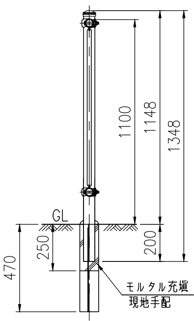
基礎杭 詳細図 (1/10)
