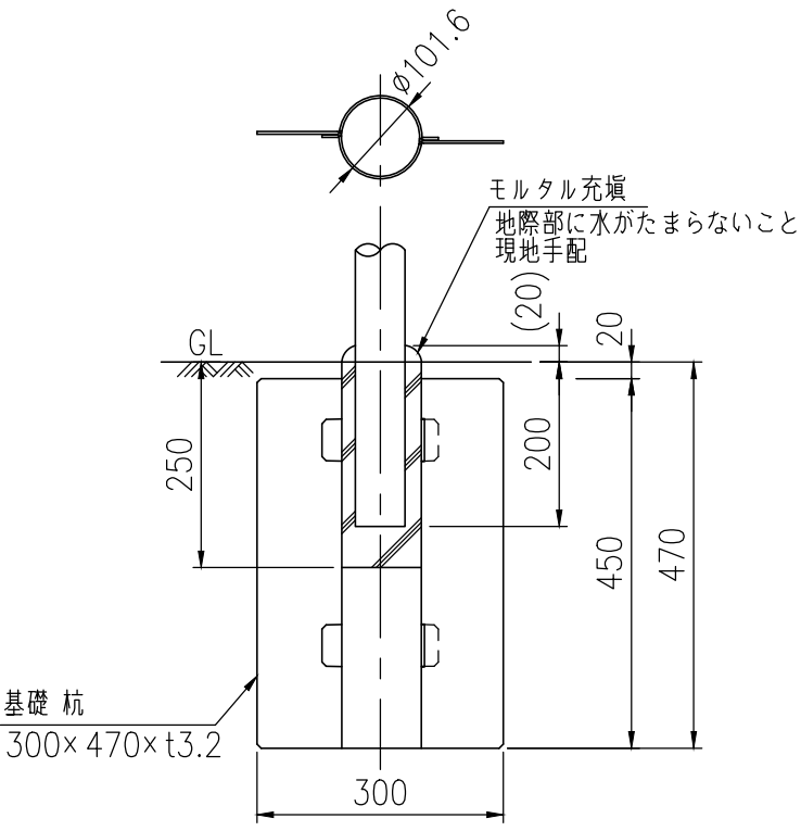
基礎杭 詳細図 (1/10)
