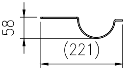
基礎杭 詳細図 (1/10)
