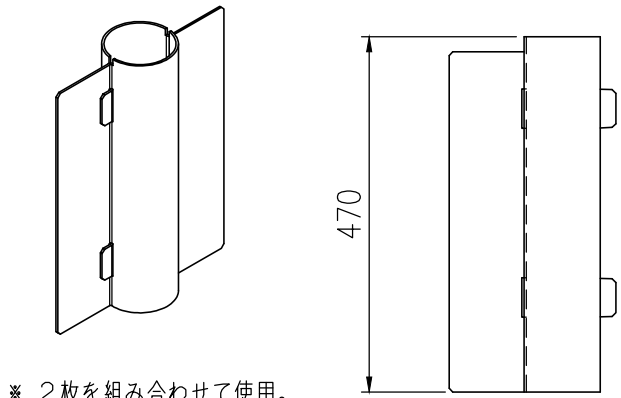
基礎杭 詳細図 (1/10)
