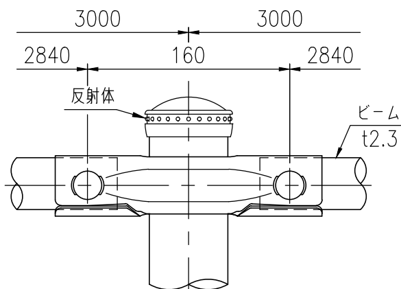
取付部詳細図 (1/4)
