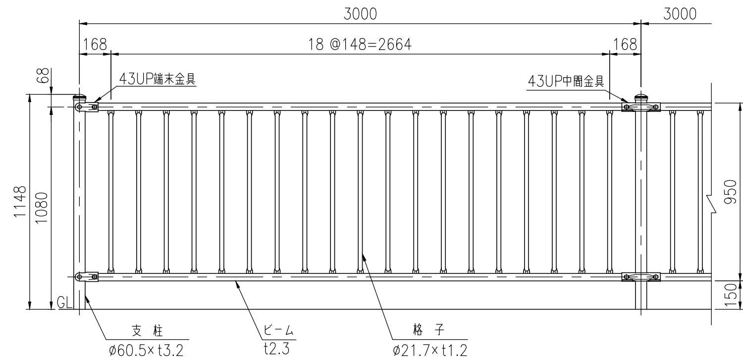
設置図 (1/20)
