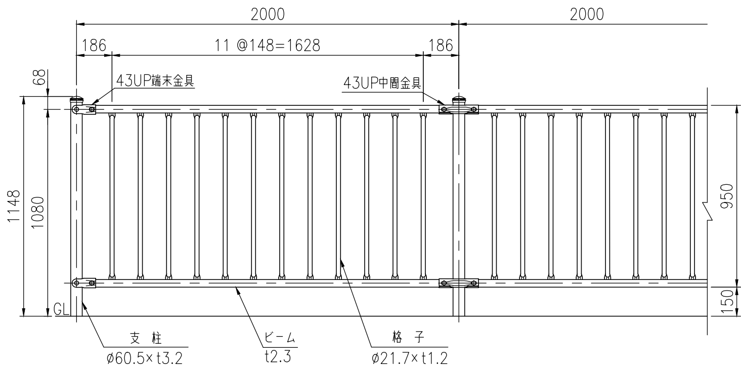
設置図 (1/20)
