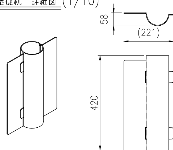
基礎杭 詳細図 (1/10)
