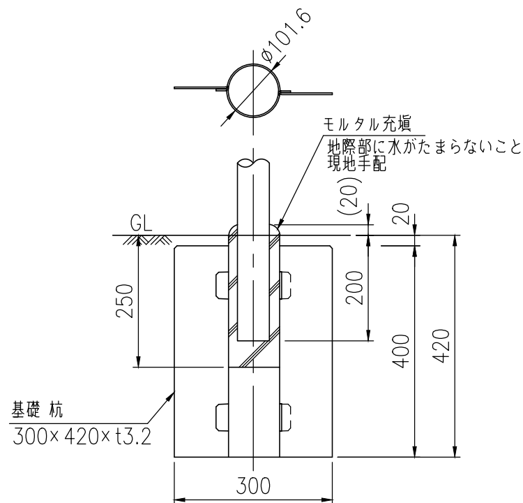
基礎部納まり 詳細図 (1/10)
