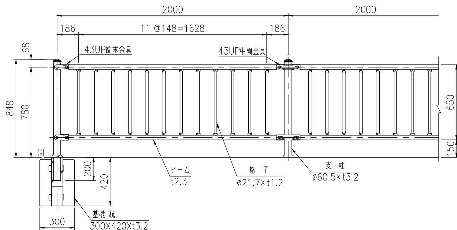
FXTC-208W20(簡易基礎杭仕様)
