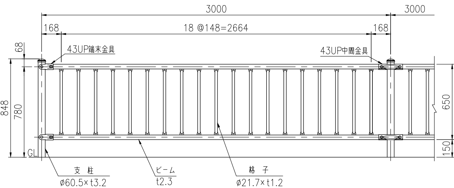
設置図 (1/20)
