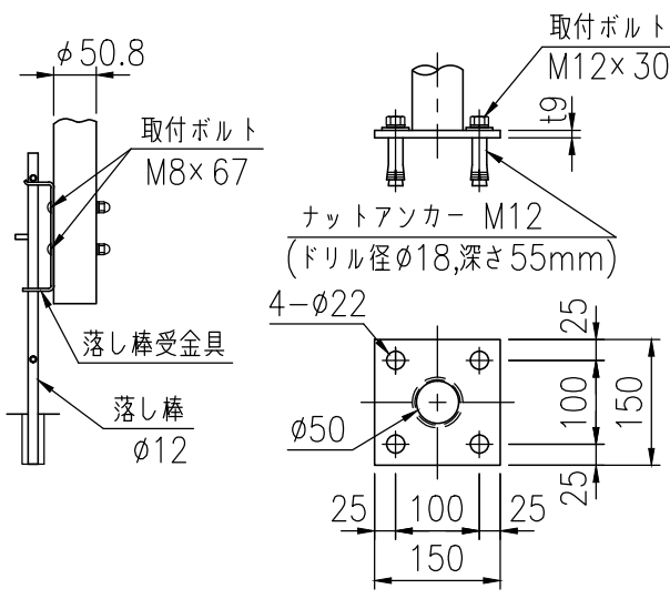
落し棒詳細図 (1/10)
