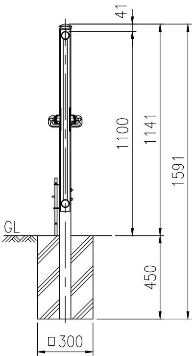
落し棒詳細図 (1/10)
