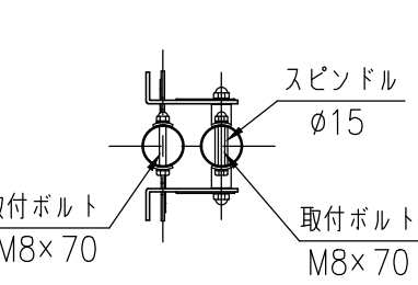
A-A断面図 (1/10)
