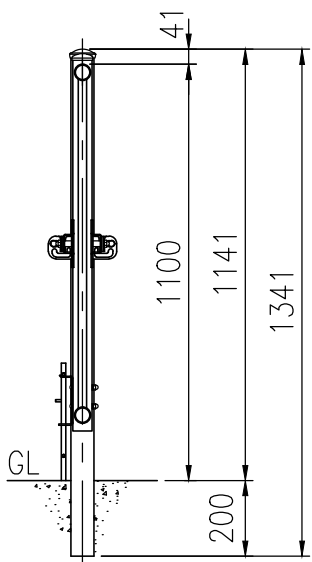
XTC-211W T-40AP111W 2.0m両開独立門扉
