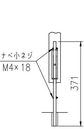
落し棒詳細図 (1/10)
