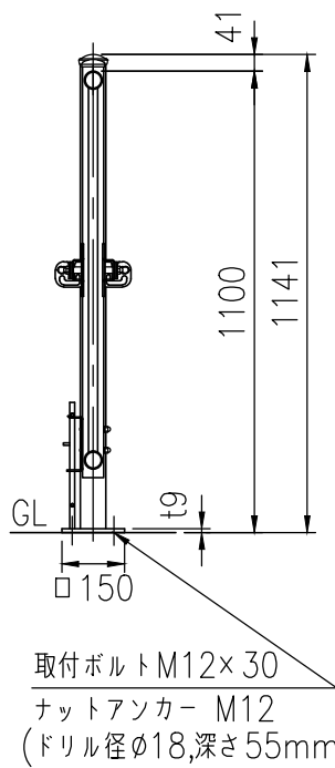
XTC-211PL T-40AP111PL 2.0m両開独立門扉
