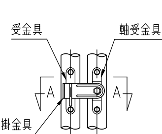
回転錠詳細図 (1/10)
