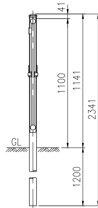
XTC-211 1.0m片開独立門扉 T-40AP111 1.0m片開独立門扉
