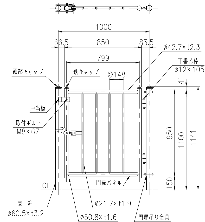
設置図 (1/20)
