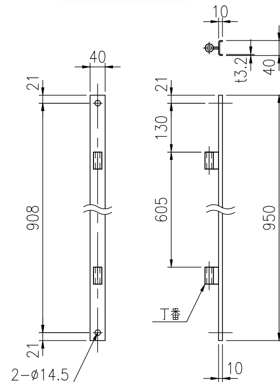
門扉吊り金具詳細図 (1/10)
