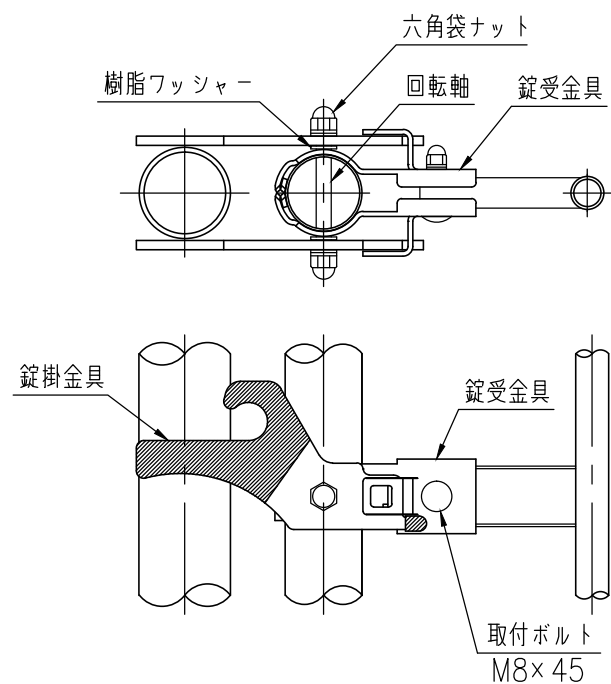
回転錠詳細図 (1/5)
