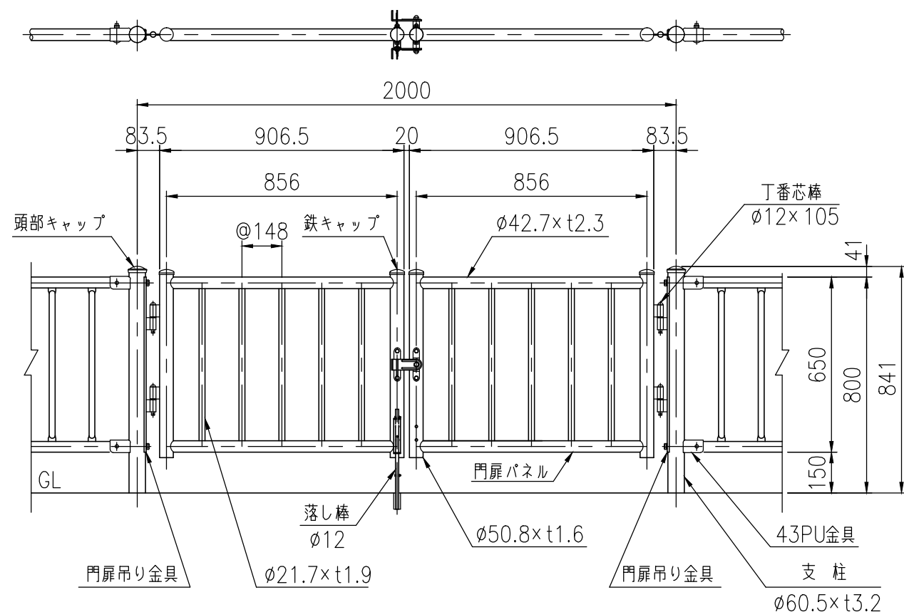
設置図 (1/20)
