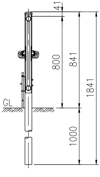
XTC-208 2.0m両開独立門扉 T-40AP81 2.0m両開独立門扉
