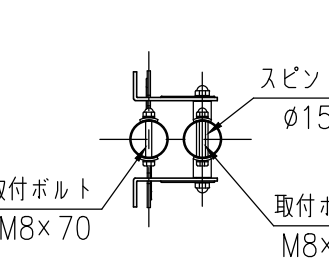
A-A断面図 (1/10)
