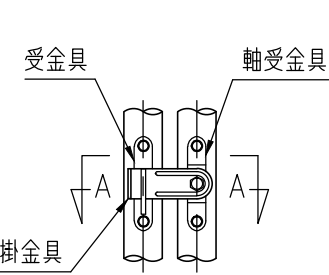
回転錠詳細図 (1/10)
