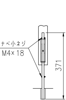
落とし棒詳細図 (1/10)
