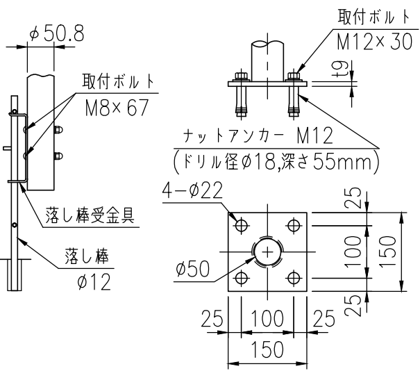
落とし棒詳細図 (1/10)
