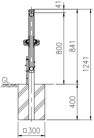
XTC-208C T-40AP81C 2.0m両開独立門扉
