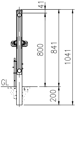
XTC-208W T-40AP81W 2.0m両開独立門扉
