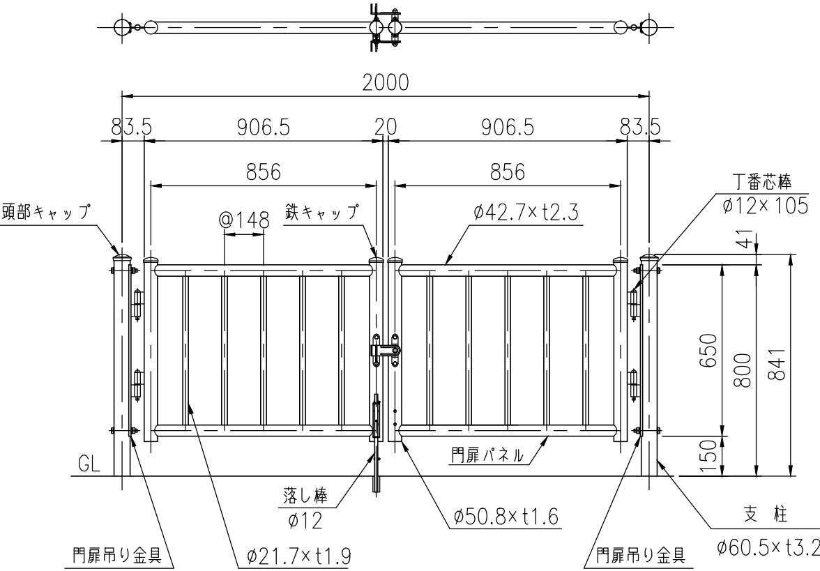
設置図 (1/20)
