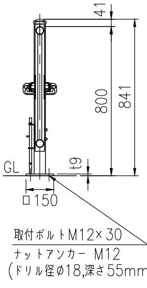
XTC-208PL T-40AP81PL 2.0m両開独立門扉
