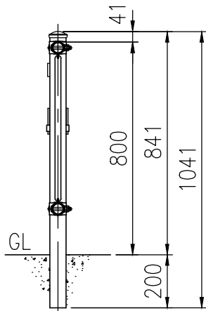
XTC-208W 1.0m片開連続門扉
