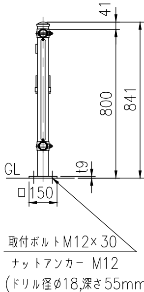
XTC-208PL 1.0m片開連続門扉
