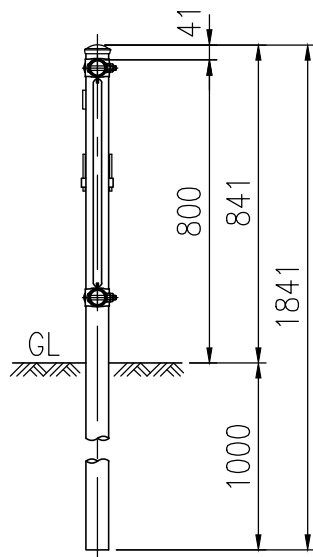
XTC-208E 1.0m片開連続門扉
