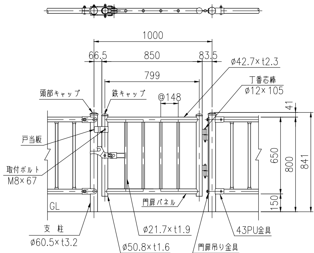
設置図 (1/20)
