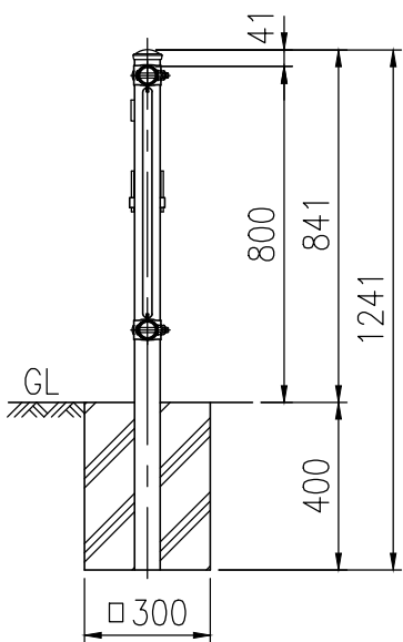
XTC-208C 1.0m片開連続門扉
