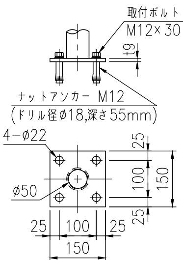
ベースプレート詳細図 (1/10)
