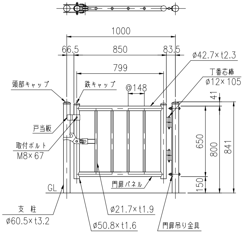
設置図 (1/20)
