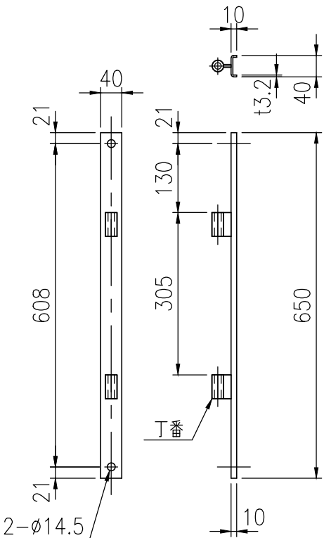
門扉吊り金具詳細図 (1/10)
