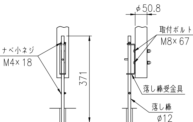
落とし棒詳細図 (1/10)
