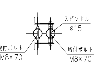
A-A断面図 (1/10)
