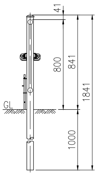
T-40AP81 2.0m両開連続門扉
