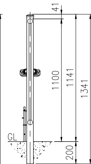
T-40AP111W 2.0m両開連続門扉
