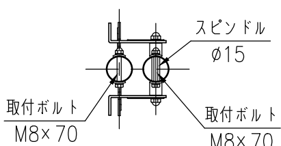
A-A断面図 (1/10)
