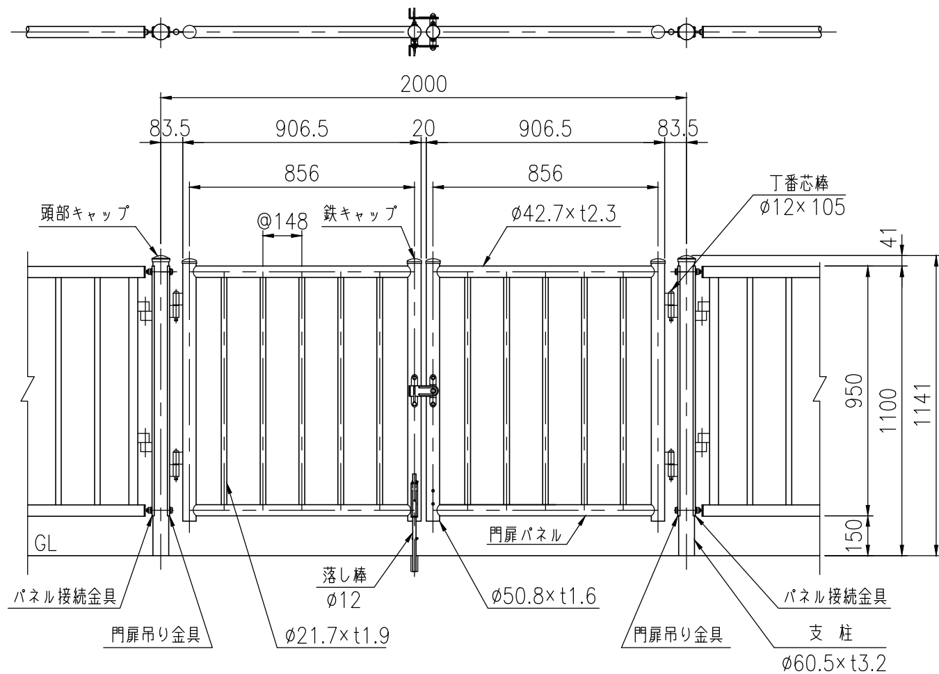
設置図 (1/20)
