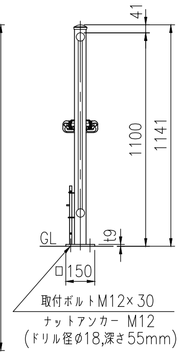
T-40AP111 2.0m両開連続門扉
