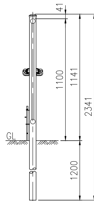
T-40AP111 2.0m両開連続門扉
