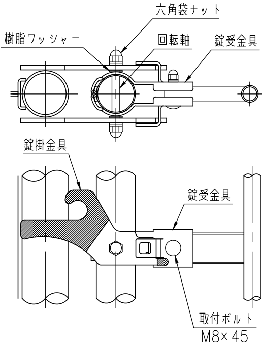
回転錠詳細図 (1/5)
