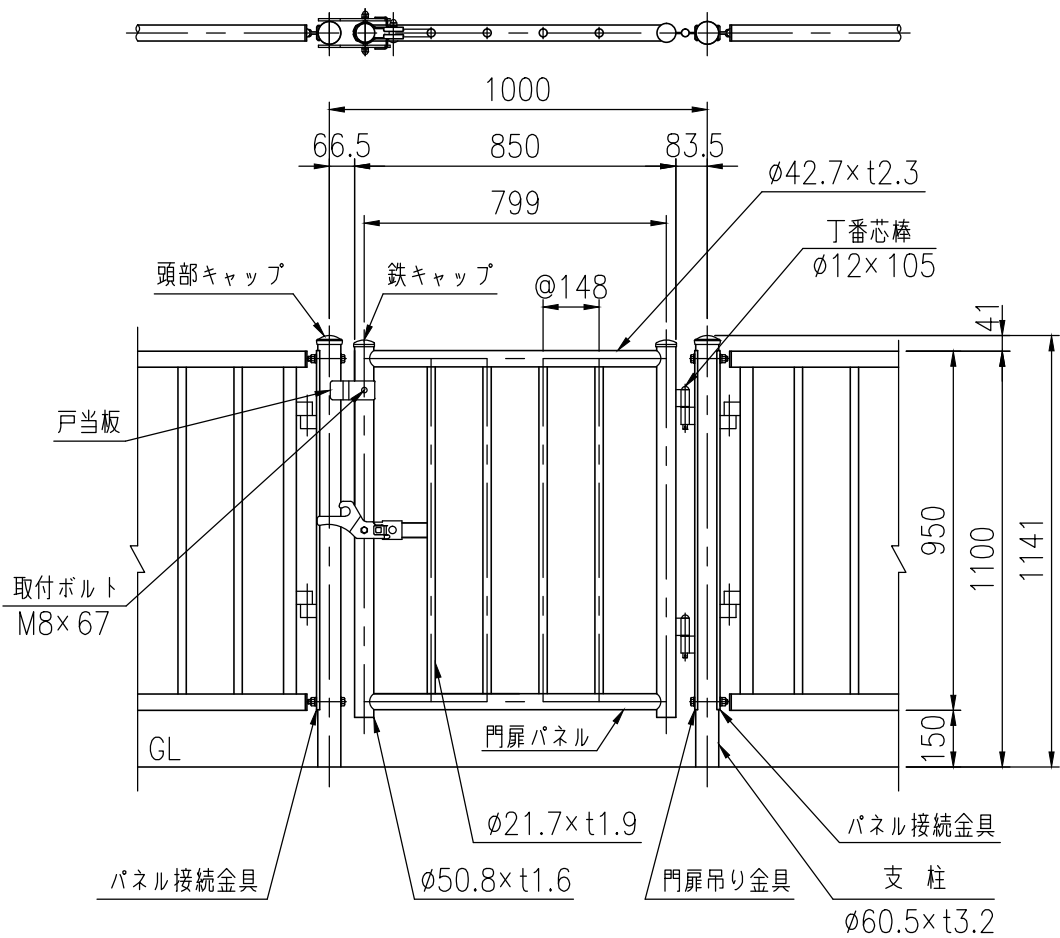
設置図 (1/20)
