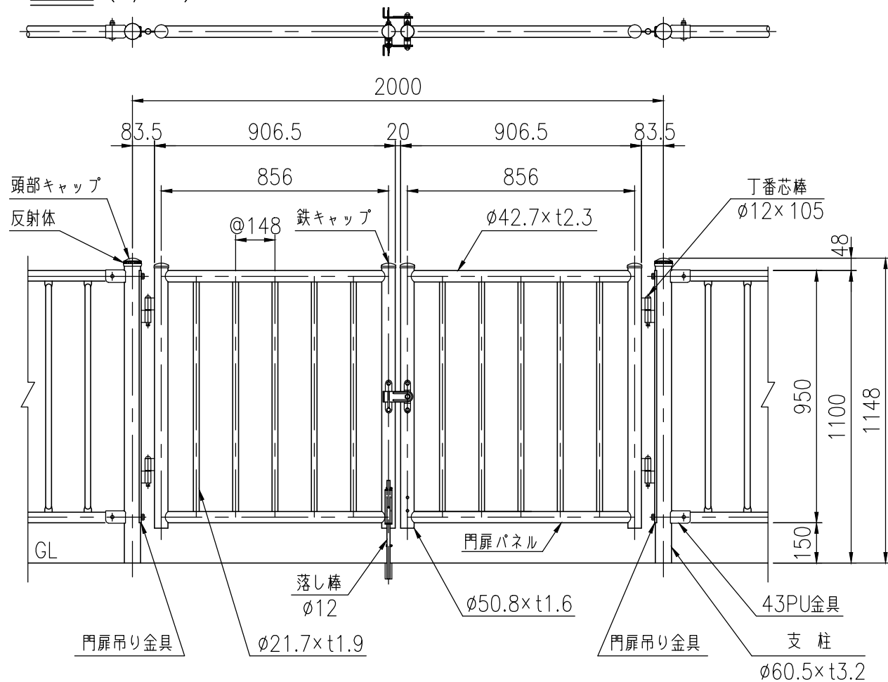
設置図 (1/20)
