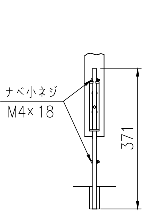
落とし棒詳細図 (1/10)
