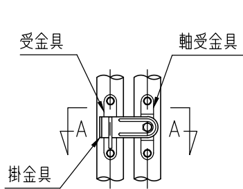
回転錠詳細図 (1/10)
