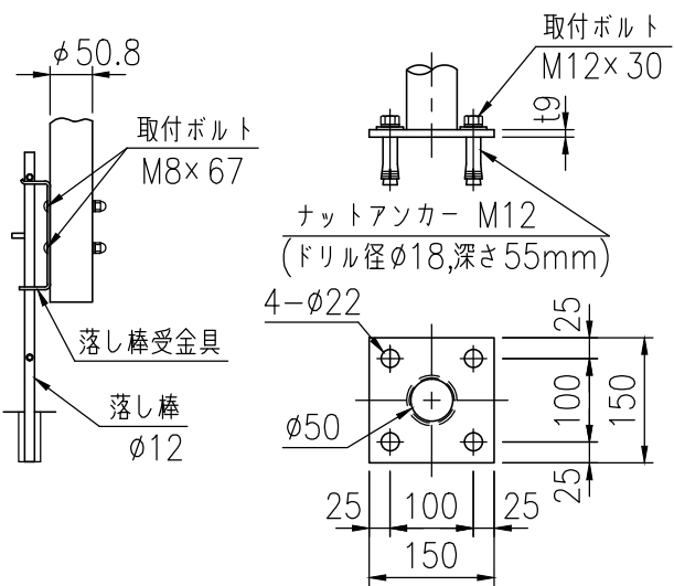
落とし棒詳細図 (1/10)
