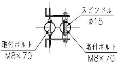
A-A断面図 (1/10)
