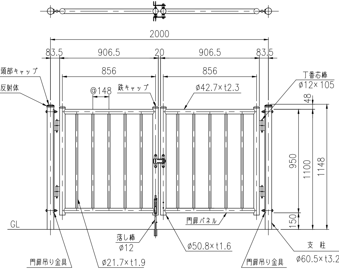
設置図 (1/20)
