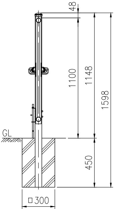
落とし棒詳細図 (1/10)
