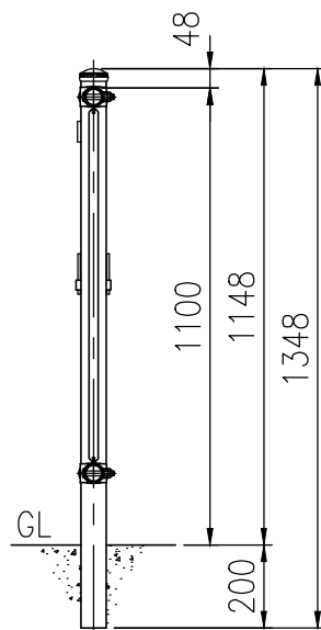
FXTC-211W 1.0m片開連続門扉
