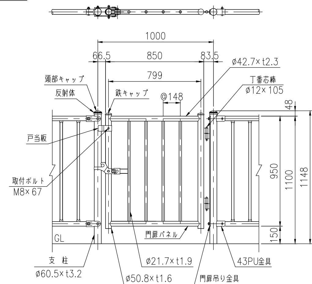
設置図 (1/20)
