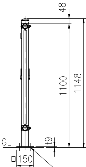
FXTC-211PL 1.0m片開連続門扉
