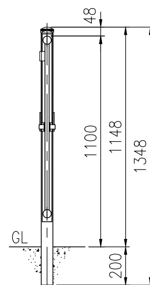
FXTC-211W FT-40AP111W 1.0m片開独立門扉
