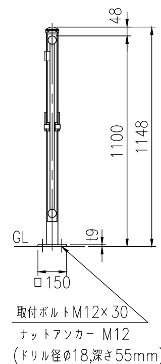
FXTC-211 1.0m片開独立門扉 FT-40AP111 1.0m片開独立門扉
