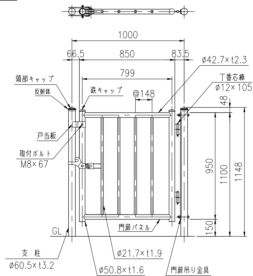
設置図 (1/20)
