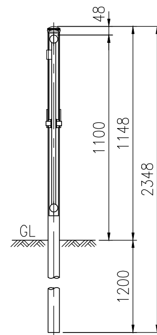
FXTC-211 1.0m片開独立門扉 FT-40AP111 1.0m片開独立門扉
