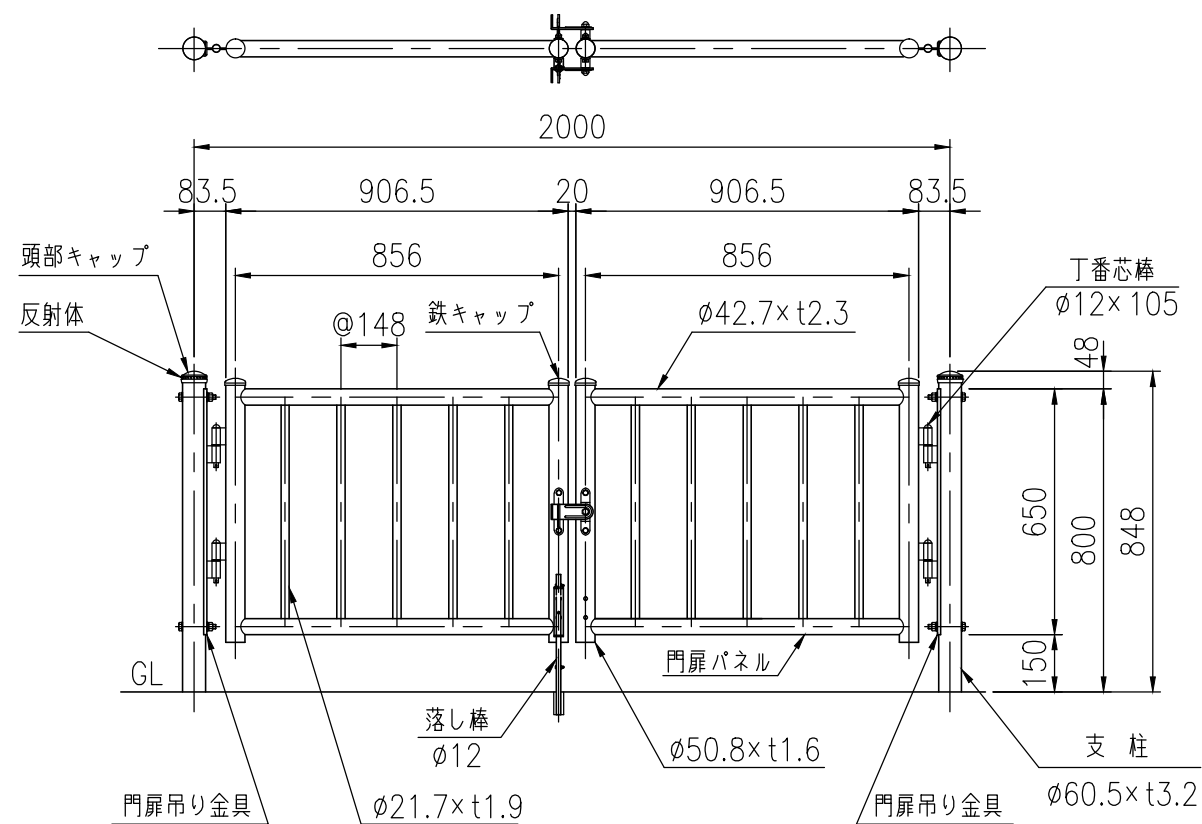
設置図 (1/20)
