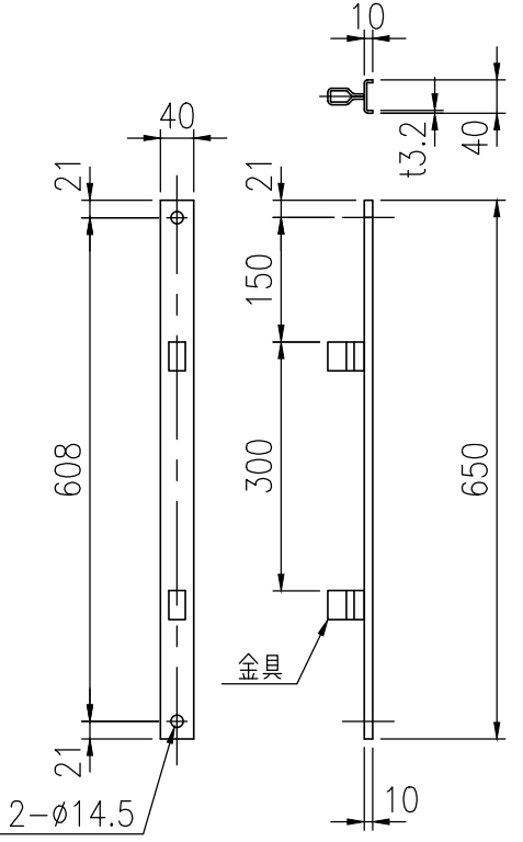
パネル接続金具詳細図 (1/10)
