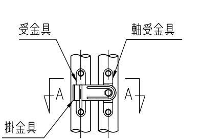
回転錠詳細図 (1/10)
