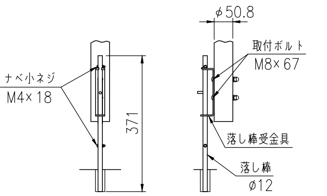
落とし棒詳細図 (1/10)
