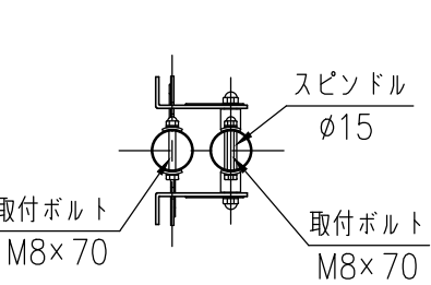
A-A断面図 (1/10)
