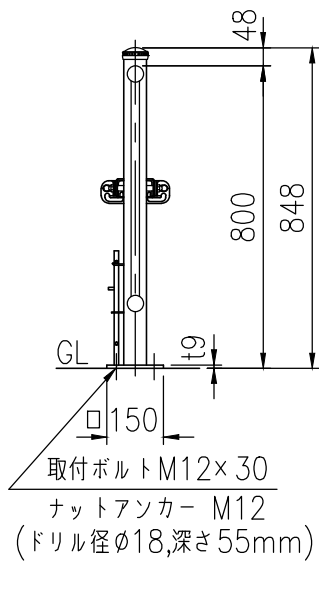
FT-40AP81 2.0m両開連続門扉
