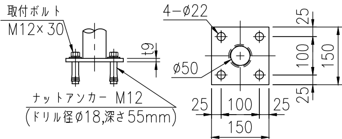
ベースプレート詳細図 (1/10)
