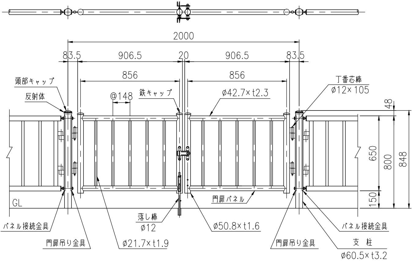
設置図 (1/20)
