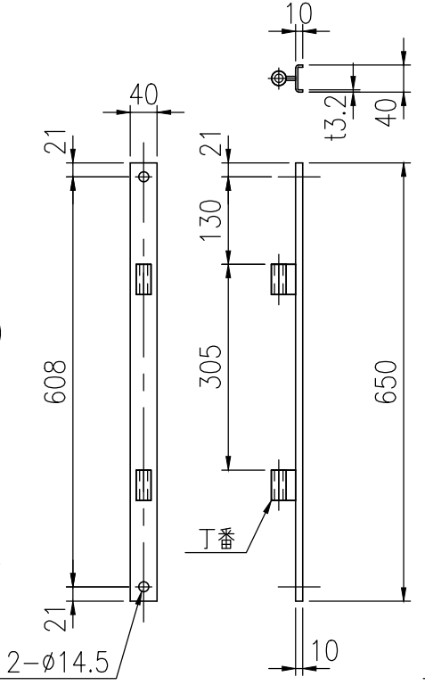
門扉吊り金具詳細図 (1/10)
