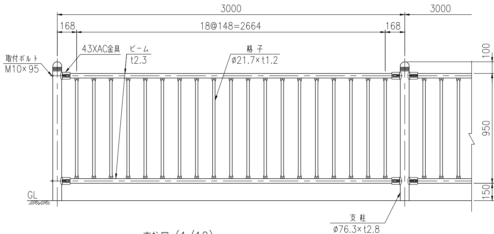
支柱図 (1/10)
