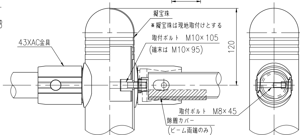
取付部詳細図 (1/3)
