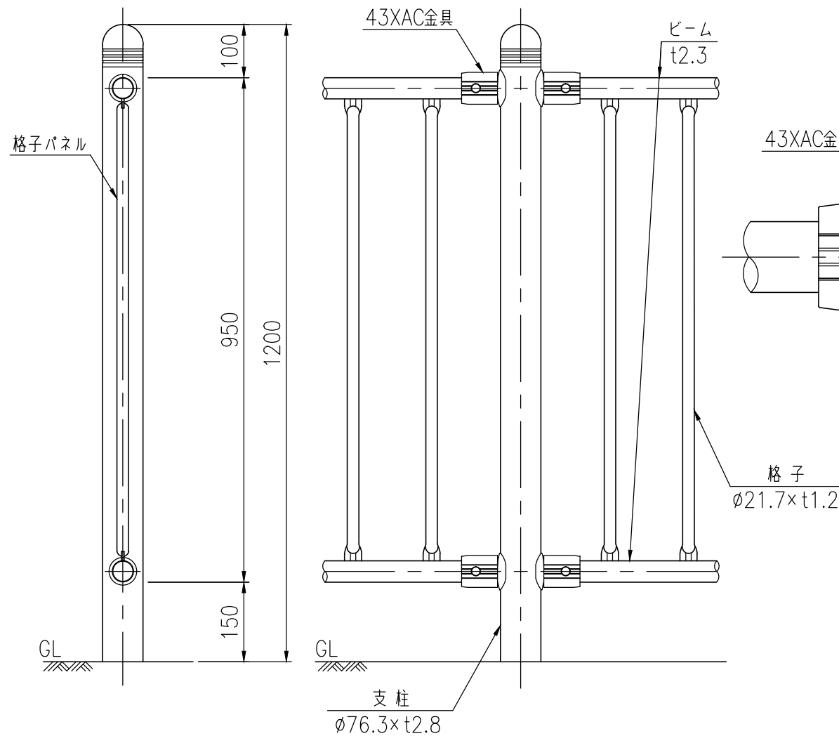
支柱図 (1/10)
