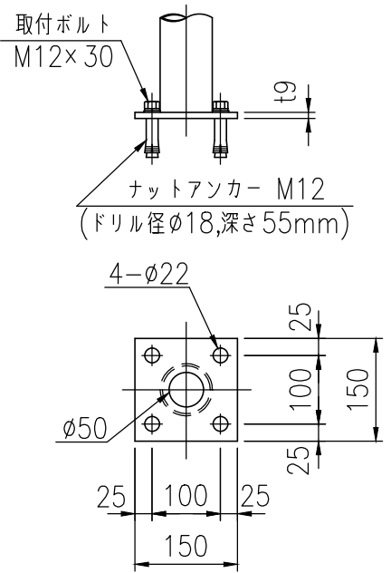
ベースプレート詳細図 (1/10)
