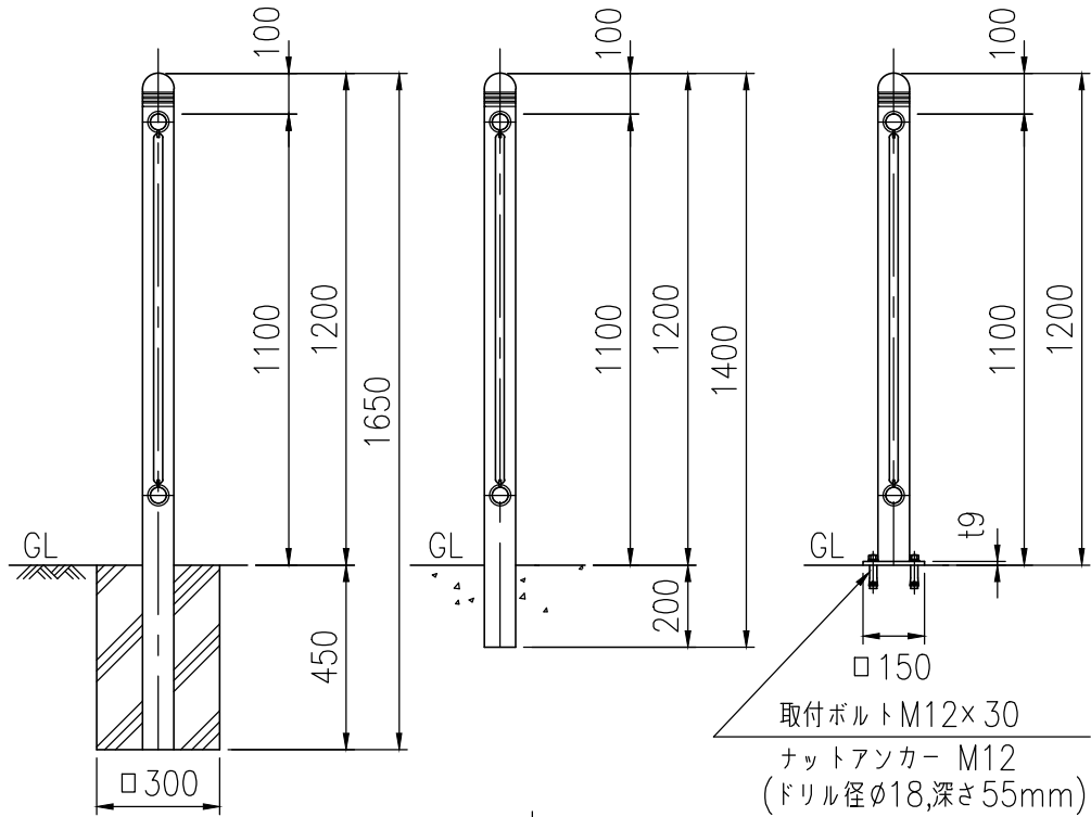
隙間カバー詳細図 (1/3)
