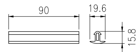
ベースプレート詳細図 (1/10)
