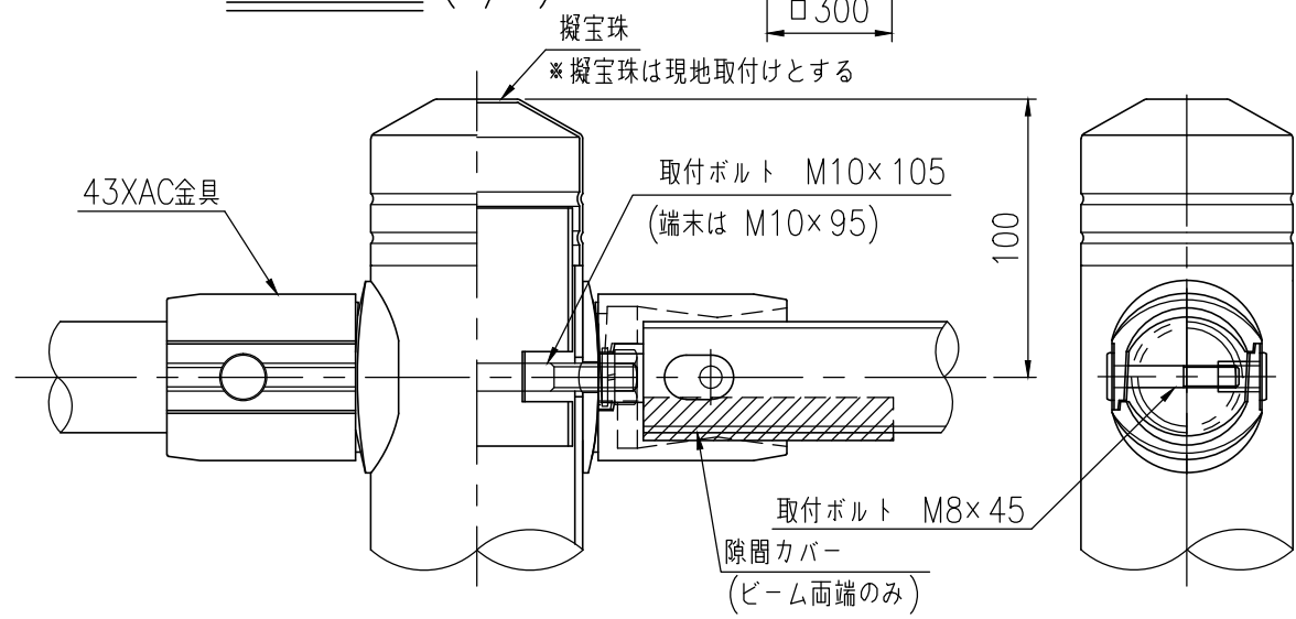
取付部詳細図 (1/3)
