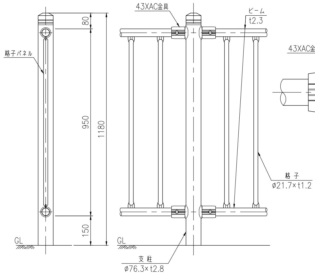
支柱図 (1/10)
