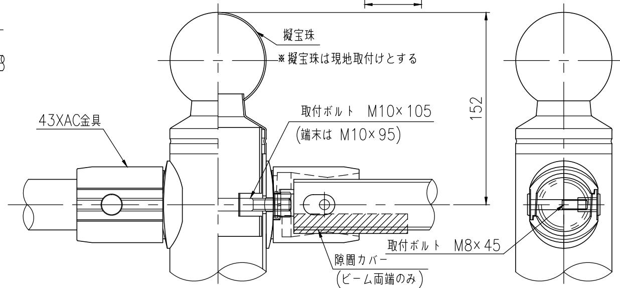
取付部詳細図 (1/3)
