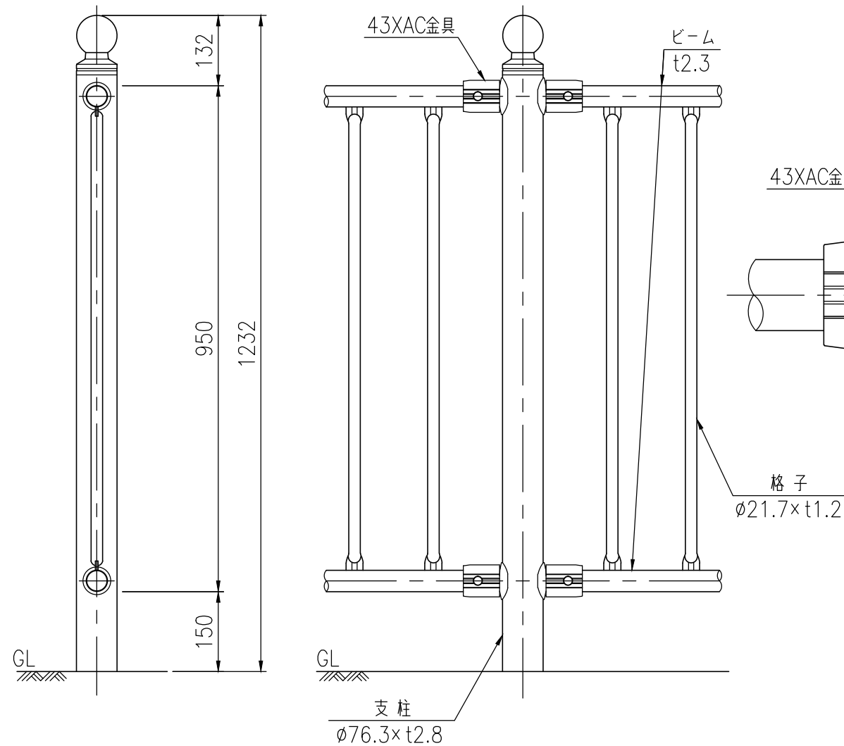
支柱図 (1/10)
